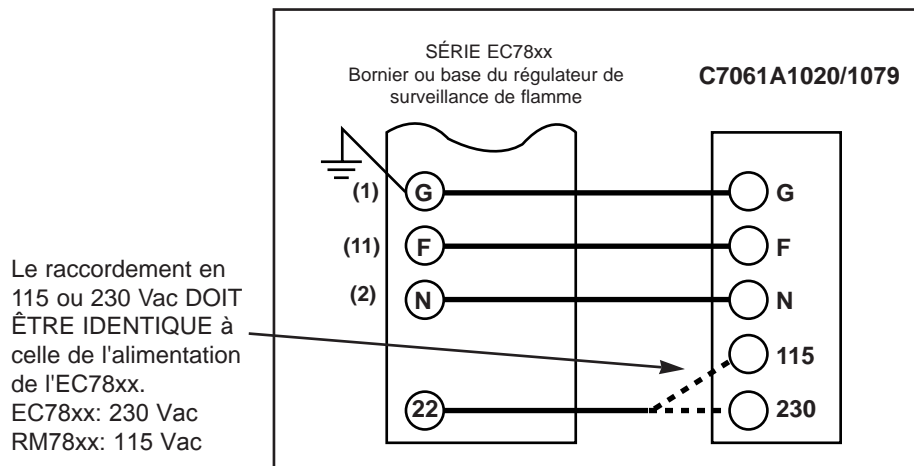
Figure 10.2 - Schéma de raccordement d'un C7061A1020/1079 avec un régulateur de surveillance de flamme Série EC/RM78xx
